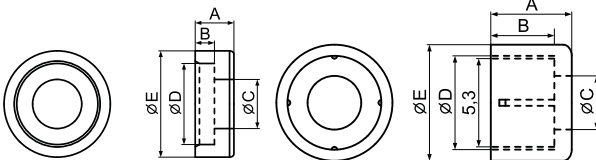
Материал: нейлон-66 Класс огнестойкости: 94V-2/94V-0 Цвет: натуральный
