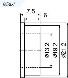
Материал: нейлон-66 Класс огнестойкости: 94V-2/94V-0 Цвет: натуральный
